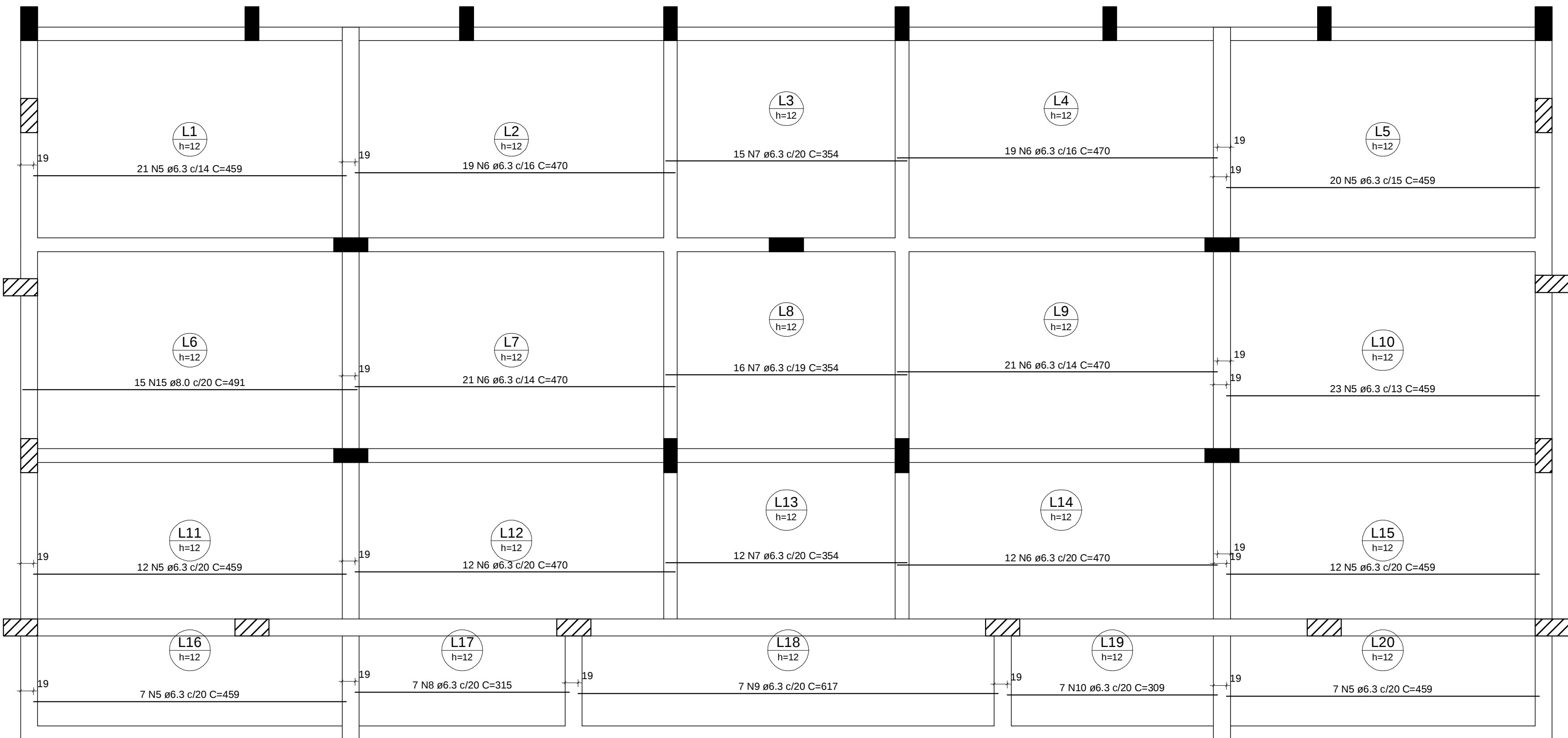
Armação positiva das lajes do pavimento Nível Inferior (Eixo X)
