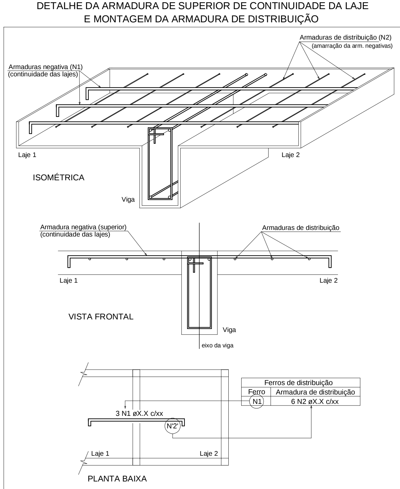
Armação negativa das lajes do pavimento Nível Inferior (Eixo Y)
