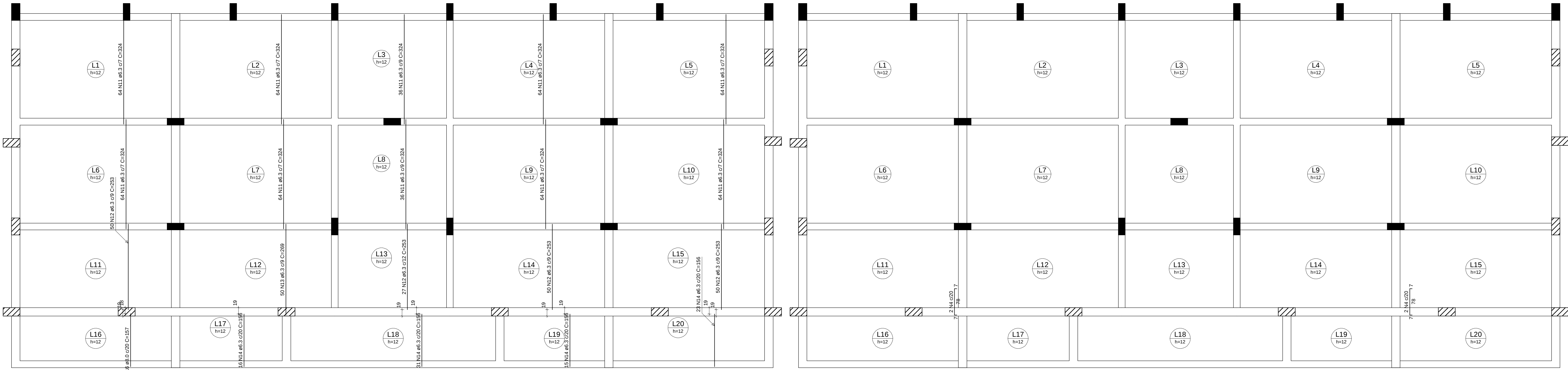
Armação positiva das lajes do pavimento Nível Inferior (Eixo Y)
