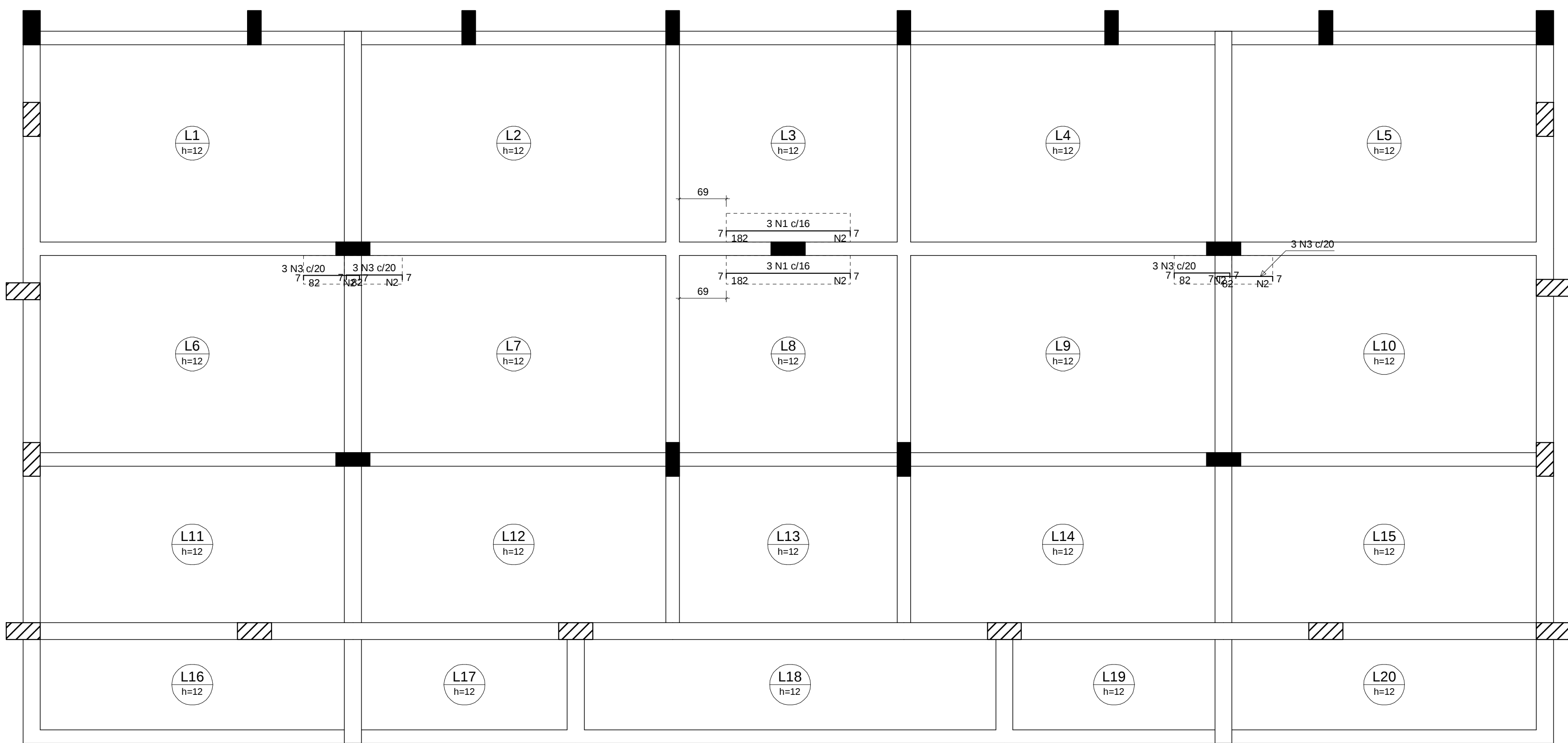
Armação negativa das lajes do pavimento Nível Inferior (Eixo X)
