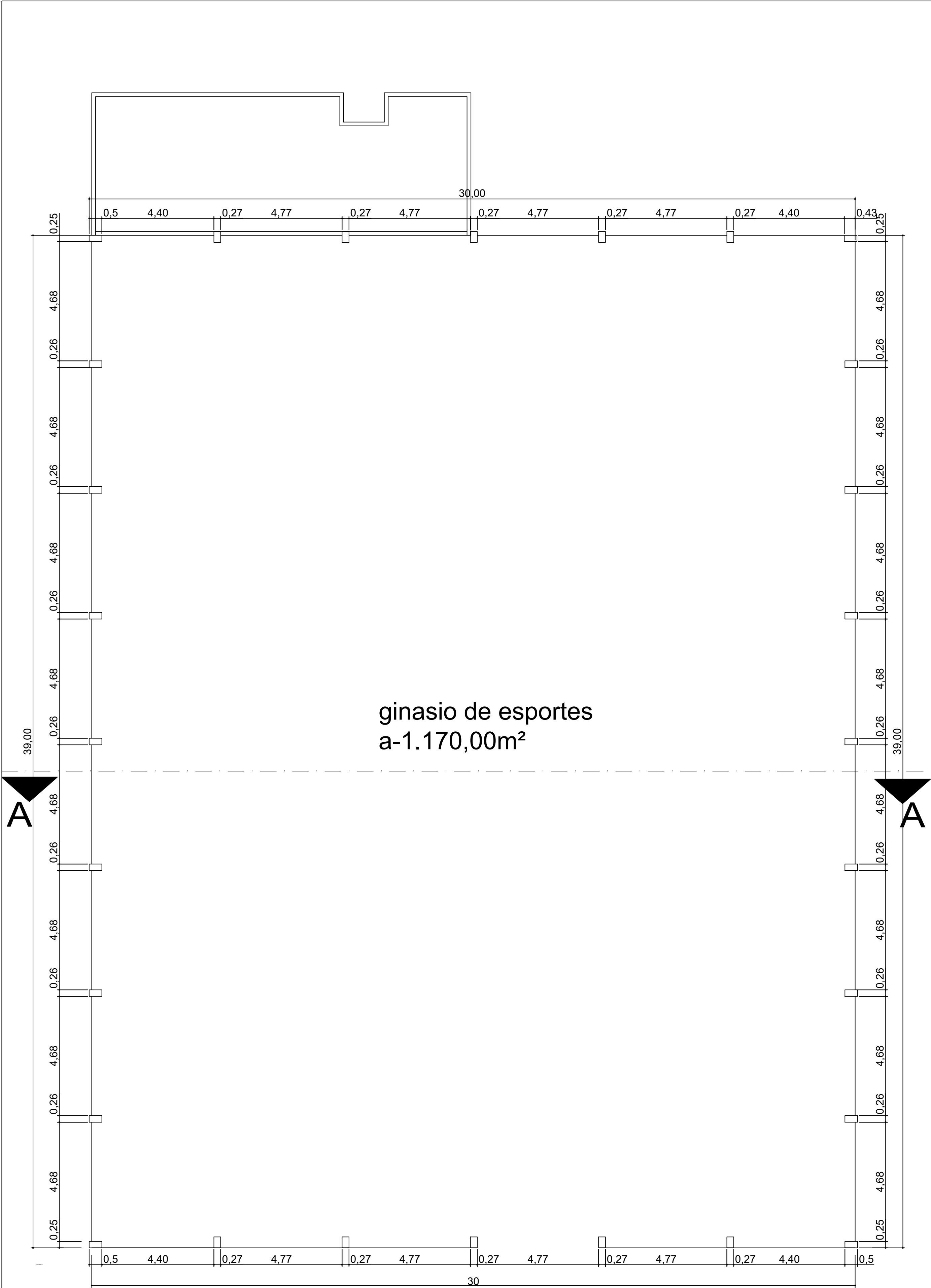
PLANTA BAIXA ESC-1/100 ÁREA =1.170,00m²
