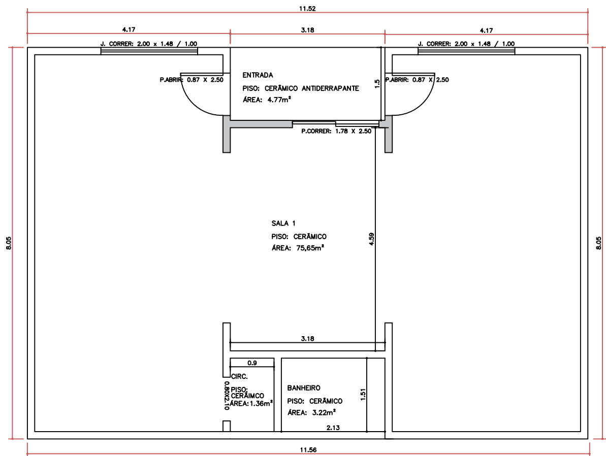
PLANTA BAIXA A=92,88m 2
